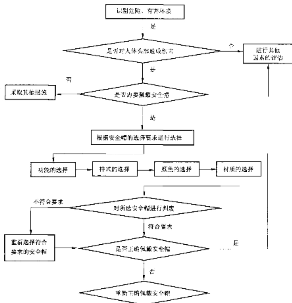
图 A.1 安全帽选用程序
